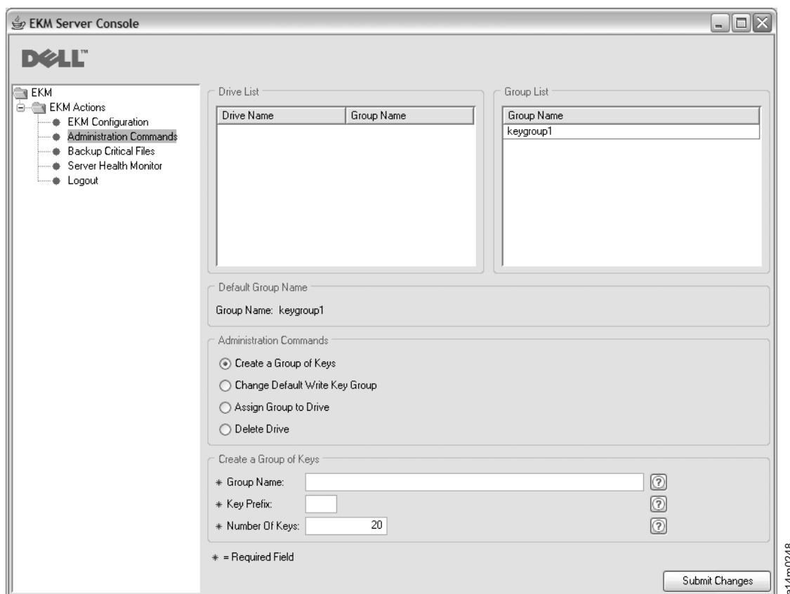
Рисунок 3-7. Create a Group of Keys (Создание группы ключей)
